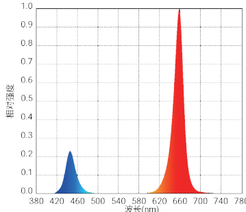
红蓝光光谱
